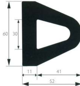
V4PD060 SEZIONE 60X52 kg/m 2 ca.
