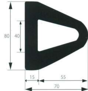
V4PD080 SEZIONE 80X70 kg/m 4 ca.
