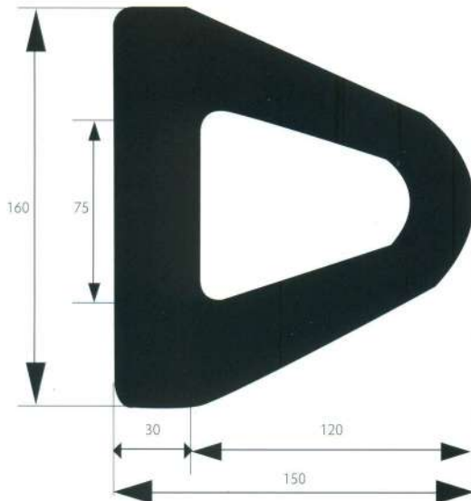
V4PD151 SEZIONE 160X150 kg/m 15,5 ca.
