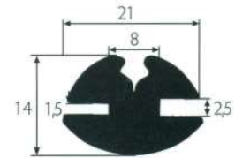
201 325 g/m con spina 260P
