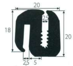
201 325 g/m con spina 260P
