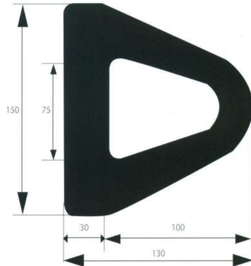
V4PD150 SEZIONE 150X130 kg/m 14 ca.
