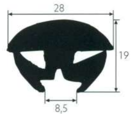
293 563 g/m con spina 205
