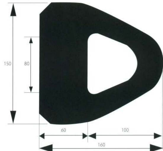
V4PD151K SEZIONE 150X160 (con smussi*) kg/m 17 ca.
