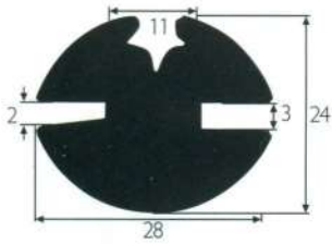
202 625 g/m con spine: 260, 205 e 206
