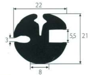
225 563 g/m con spina 260
